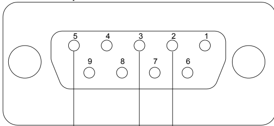
Sub-D 9 pol Stecker Ansicht Lötseite
