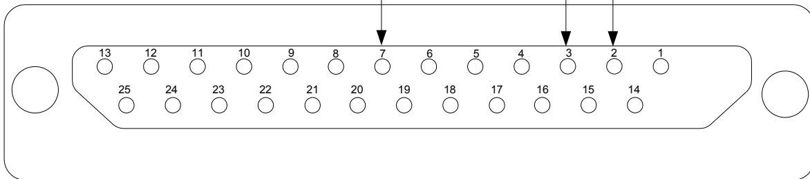
Sub-D 25 pol Stecker Ansicht Lötseite
